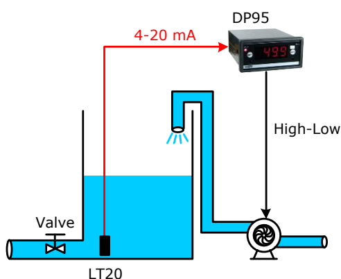
การวัดและควบคุมระดับของเหลว
