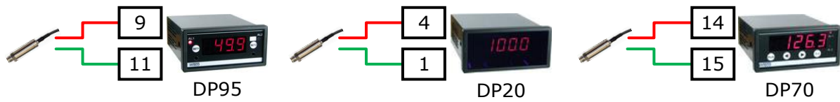
การต่อสายเข้ากับ Indicator รุ่นต่างๆของ Wisco
