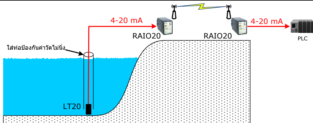
วัดระดับน้ำในแม่น้ำ
