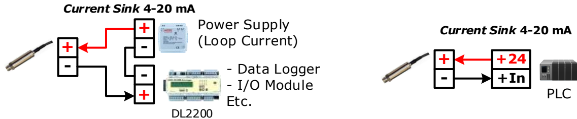
การต่อสายเข้ากับ Indicator รุ่นต่างๆของ Wisco
